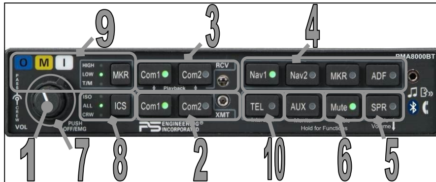
PMA8000BT controls
